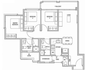
3 - Bedroom
